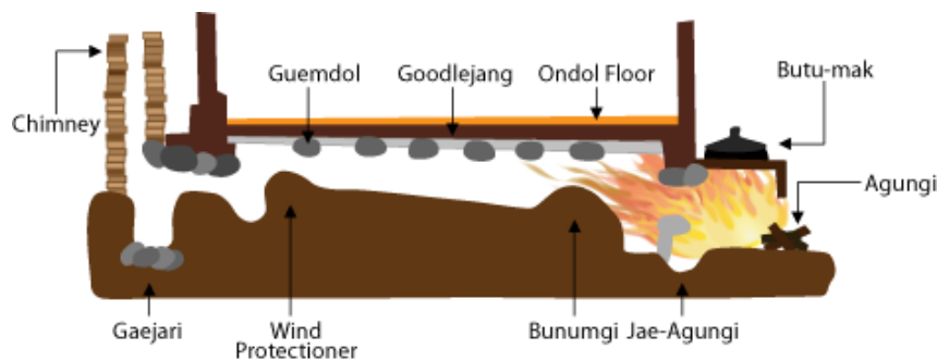
전통 온돌의 구조
